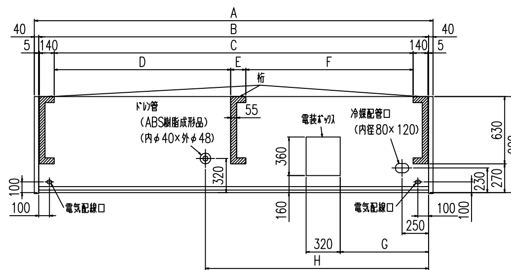
平面図
