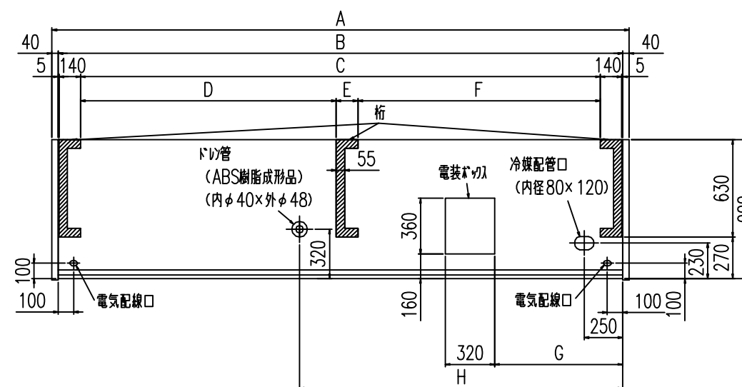
平面図
