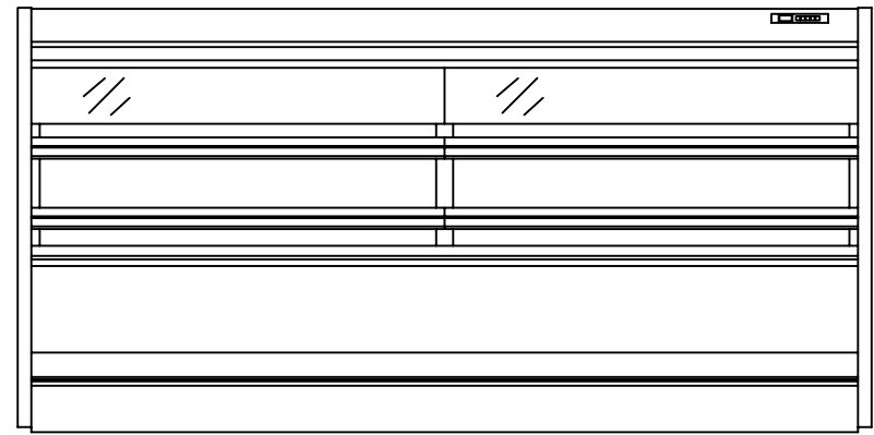
(8尺 S=1/25) 正面図
