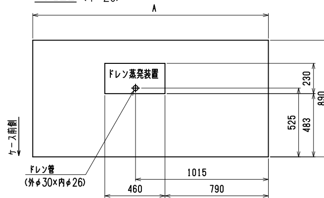
排水位置図 (1/20)
