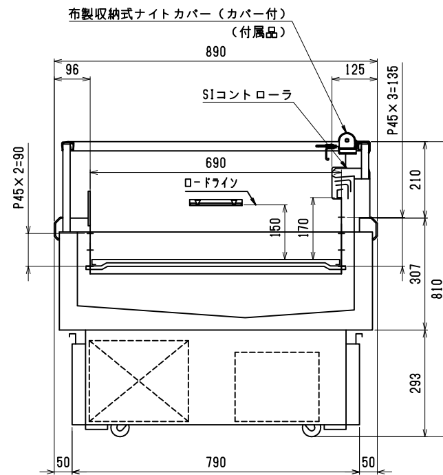
排水位置図 (1/20)
