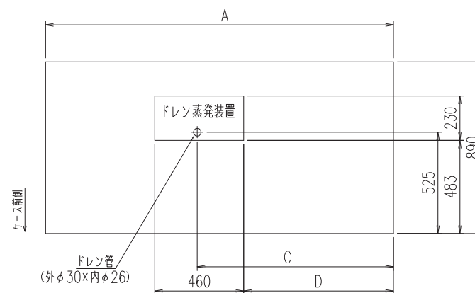
排水位置図 (1/20)
