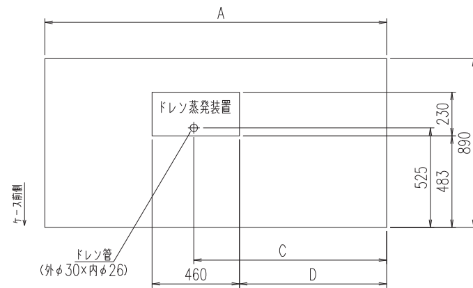
排水位置図 (1/20)
