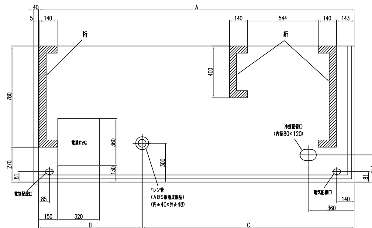
底部平面図
