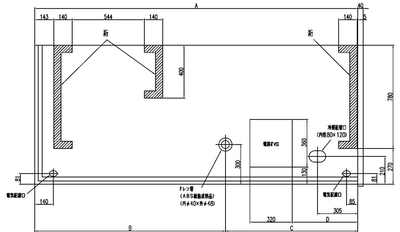
底部平面図
