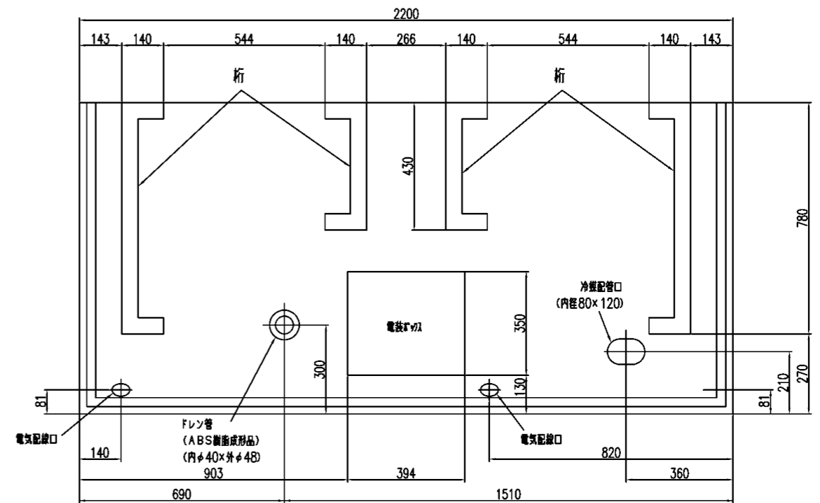
底部平面図
