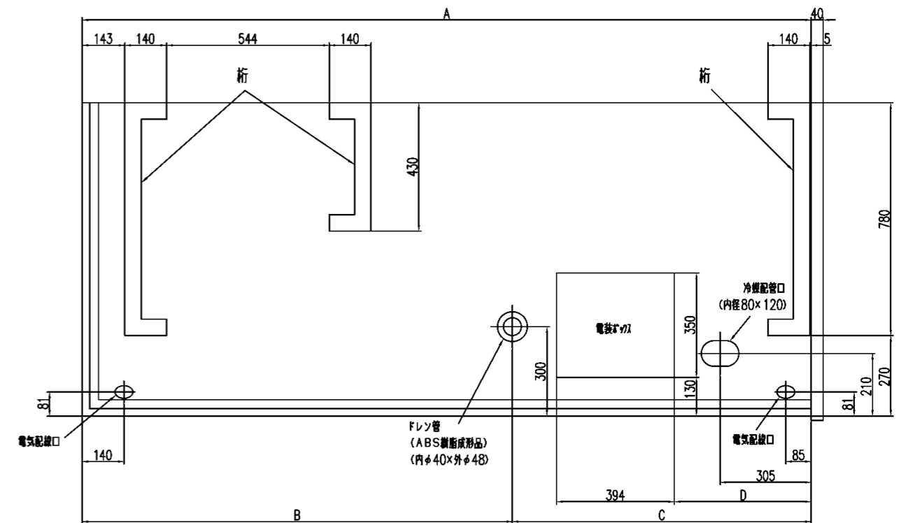
底部平面図
