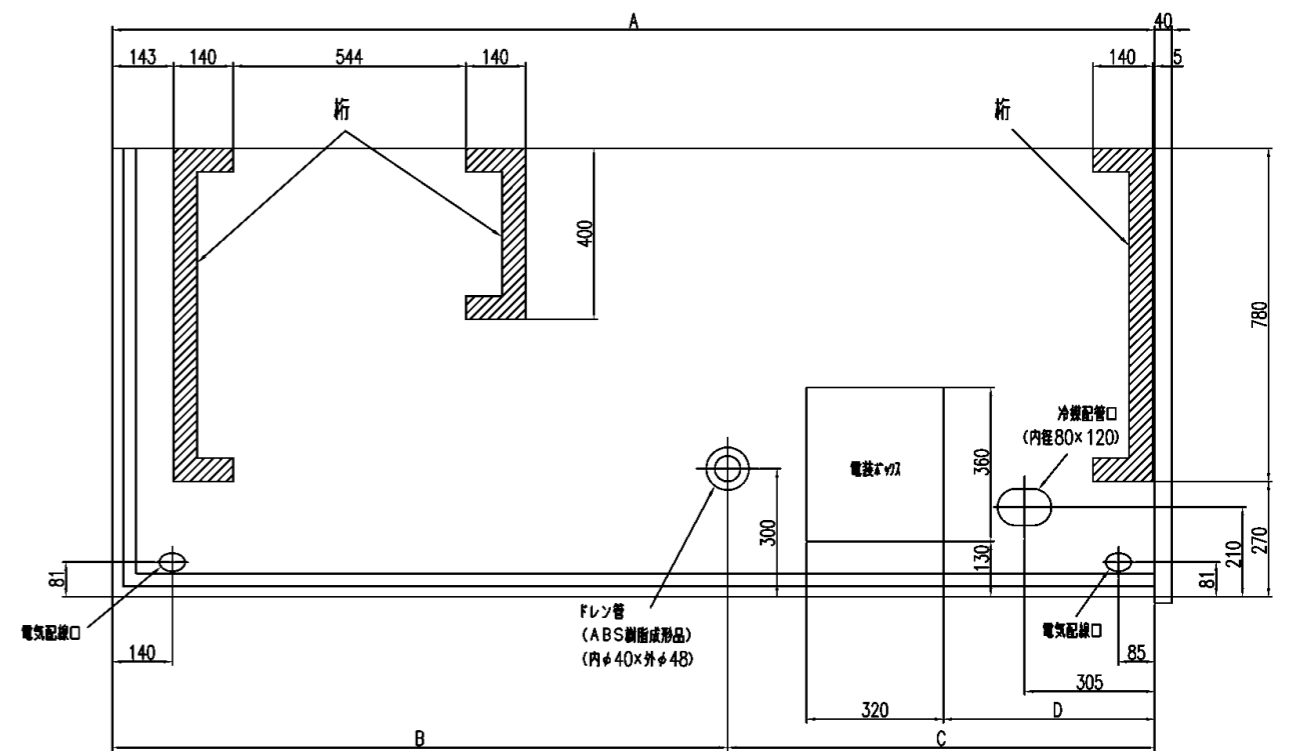
底部平面図
