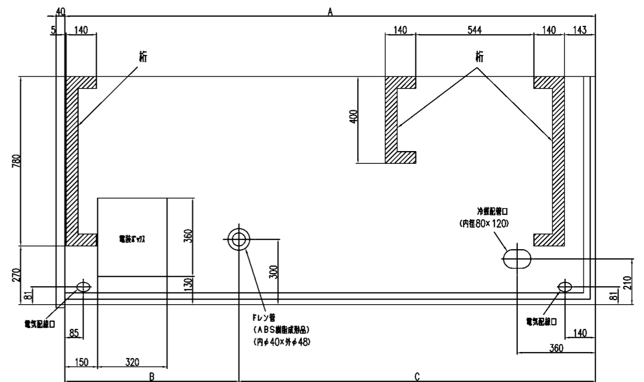
底部平面図
