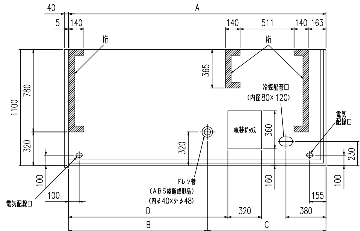
平面図
