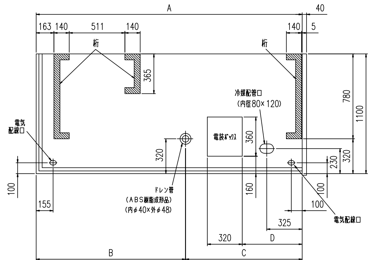
平面図
