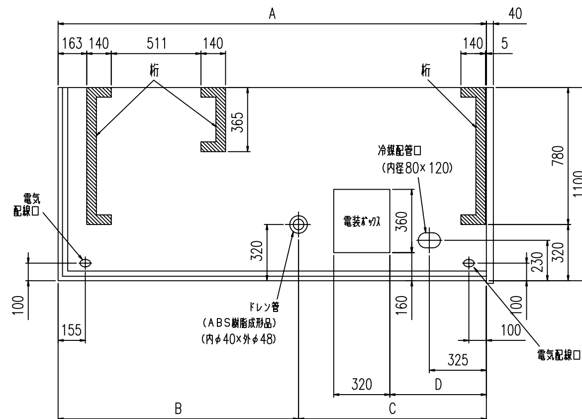
平面図
