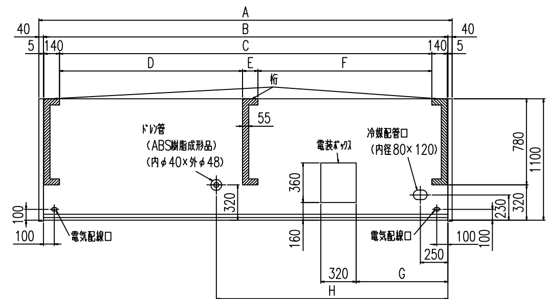
平面図
