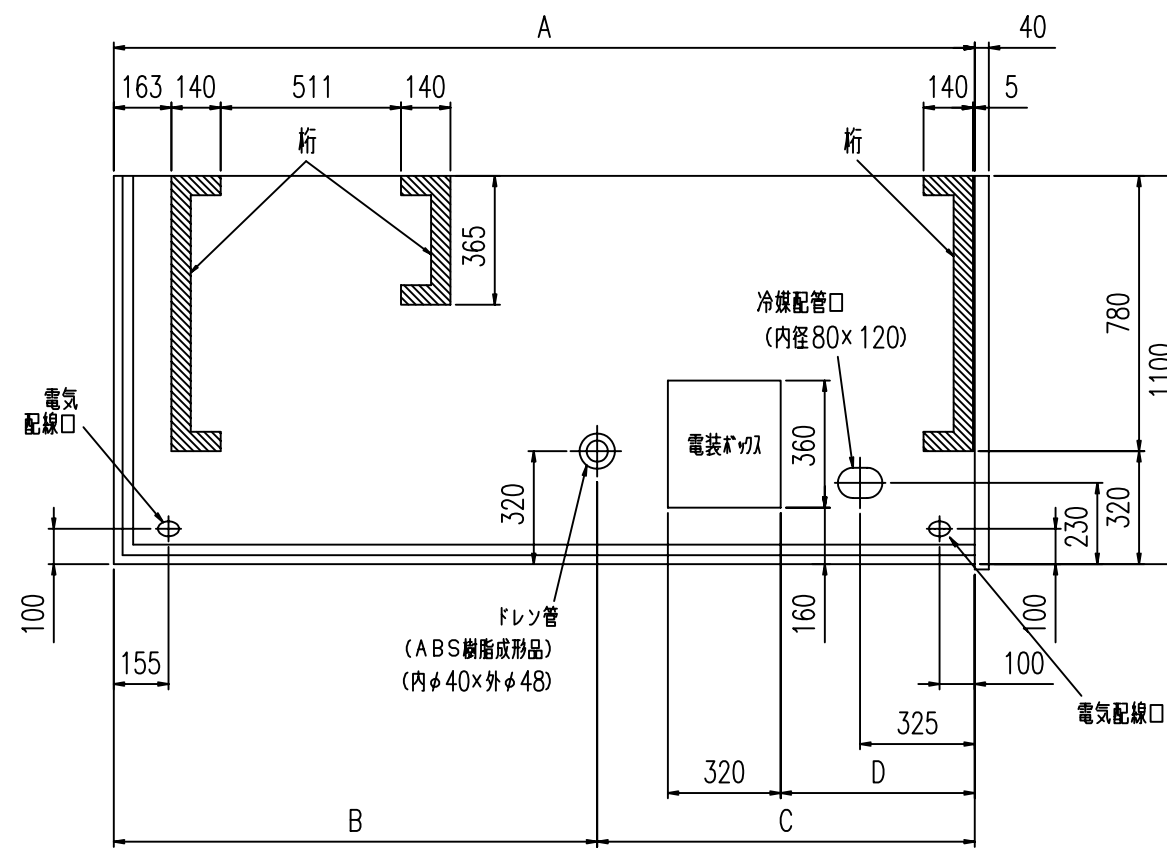
平面図
