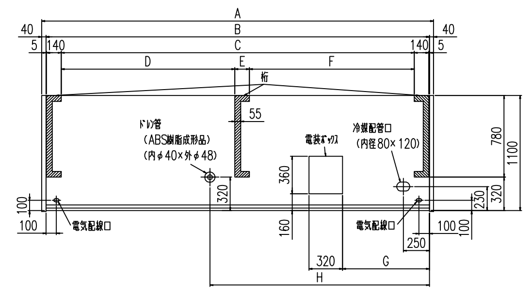
平面図
