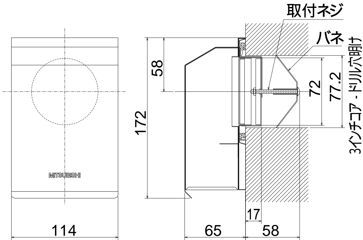
防虫網詳細図
