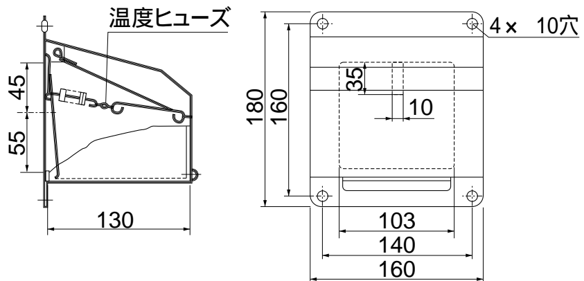
板厚:閉鎖部1.5mm ウェザーカバー部0.8mm (単位mm)
