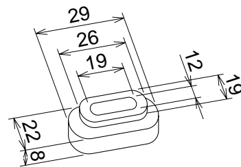
ゴムブッシュ詳細図
