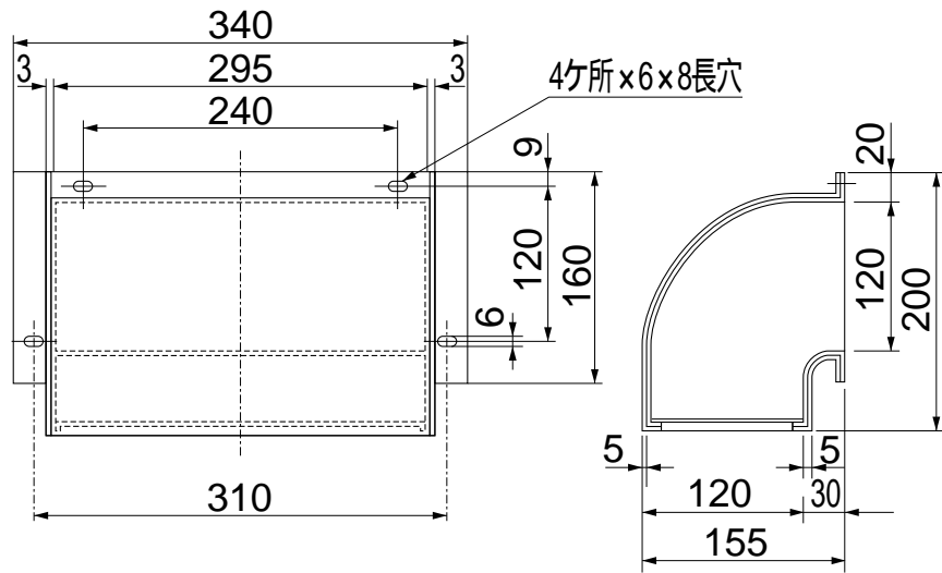
金網詳細図
