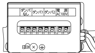
結線部(回路ケ-ス側面)
