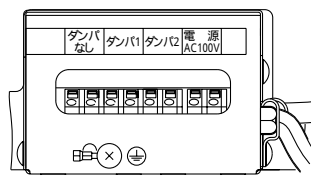
結線部(回路ケ-ス側面)
