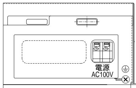
結線部(回路ケ-ス)
