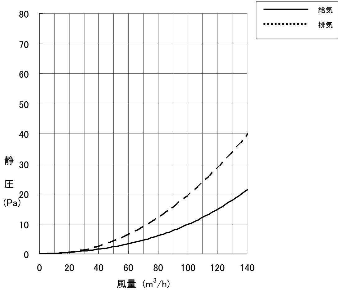
P-200K-BN , P-200KBN2 圧損特性
