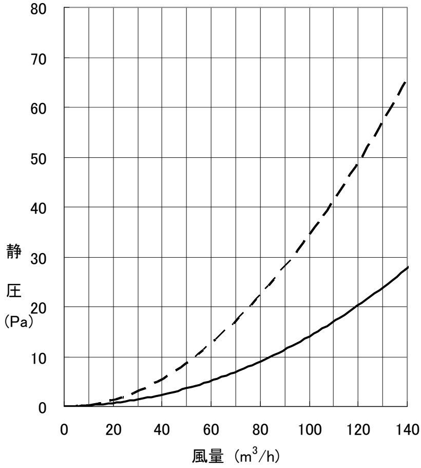
P-200K-CVD , P-200KCVD2 压損特性
