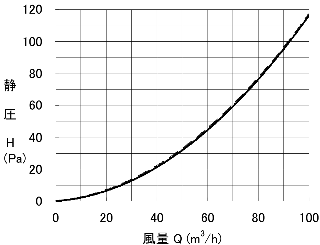
P-50VSSQ 5 圧損特性 [適用パイプ φ100二層管]
