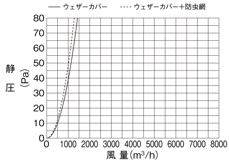
防火ダンパー付タイプ(排気)
