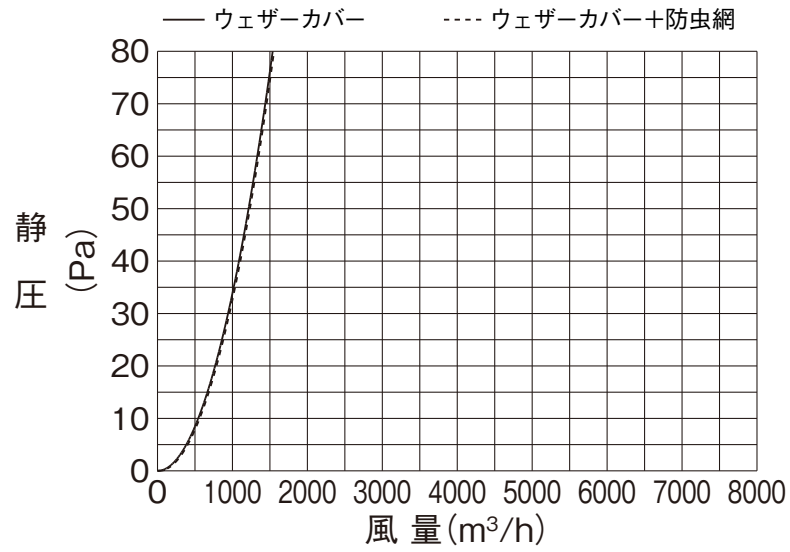
防火ダンパー付タイプ(給気)
