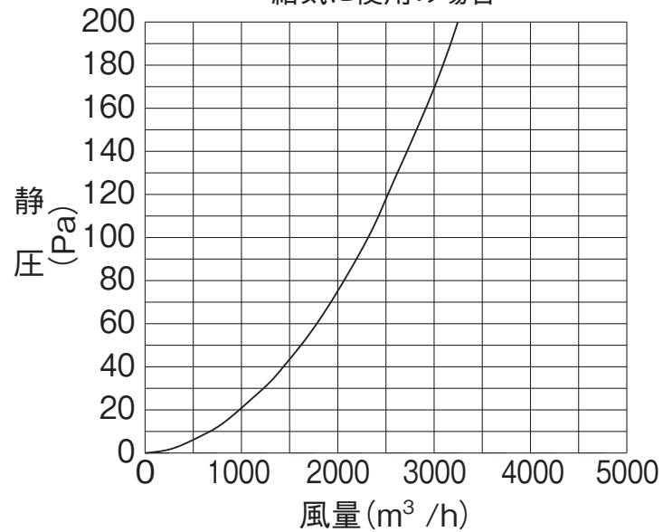
給気に使用の場合
