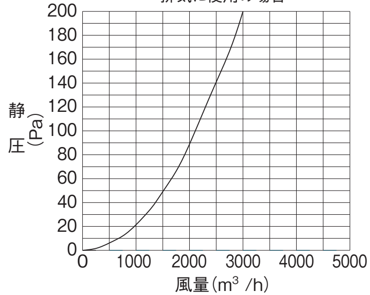
排気に使用の場合
