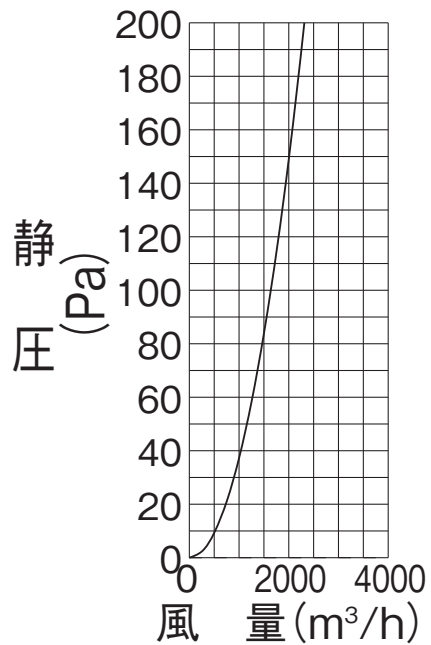
給気
