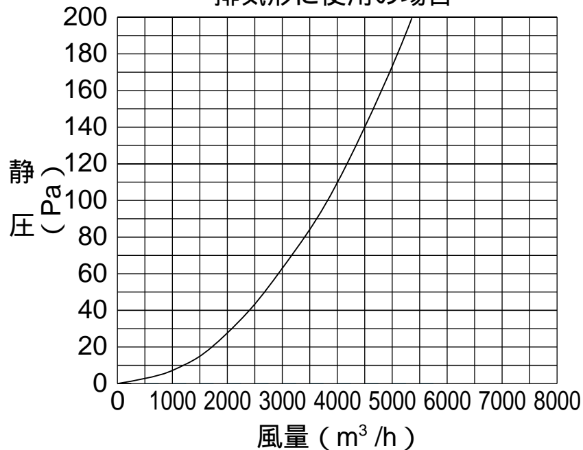
排気形に使用の場合
