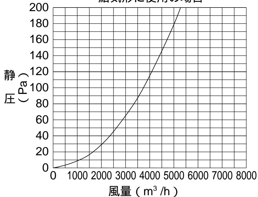
給気形に使用の場合
