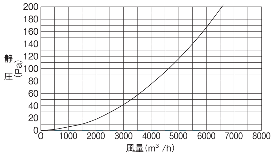
排気に使用の場合
