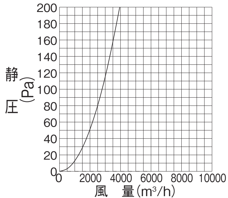
排気
