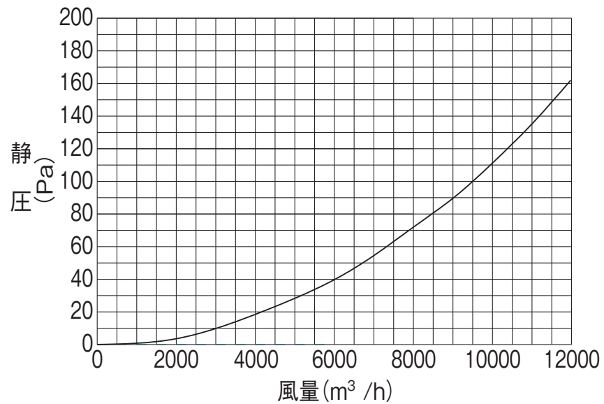
給気に使用の場合
