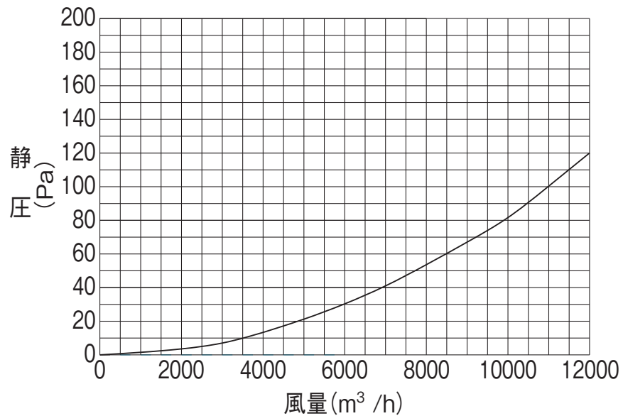
排気に使用の場合
