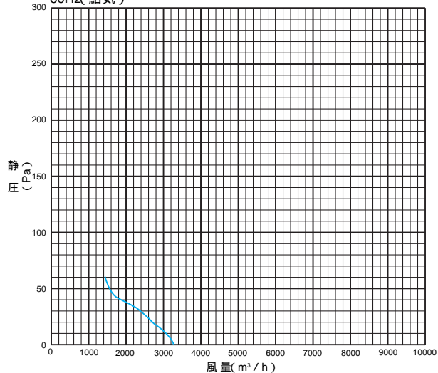
60Hz(給気)
