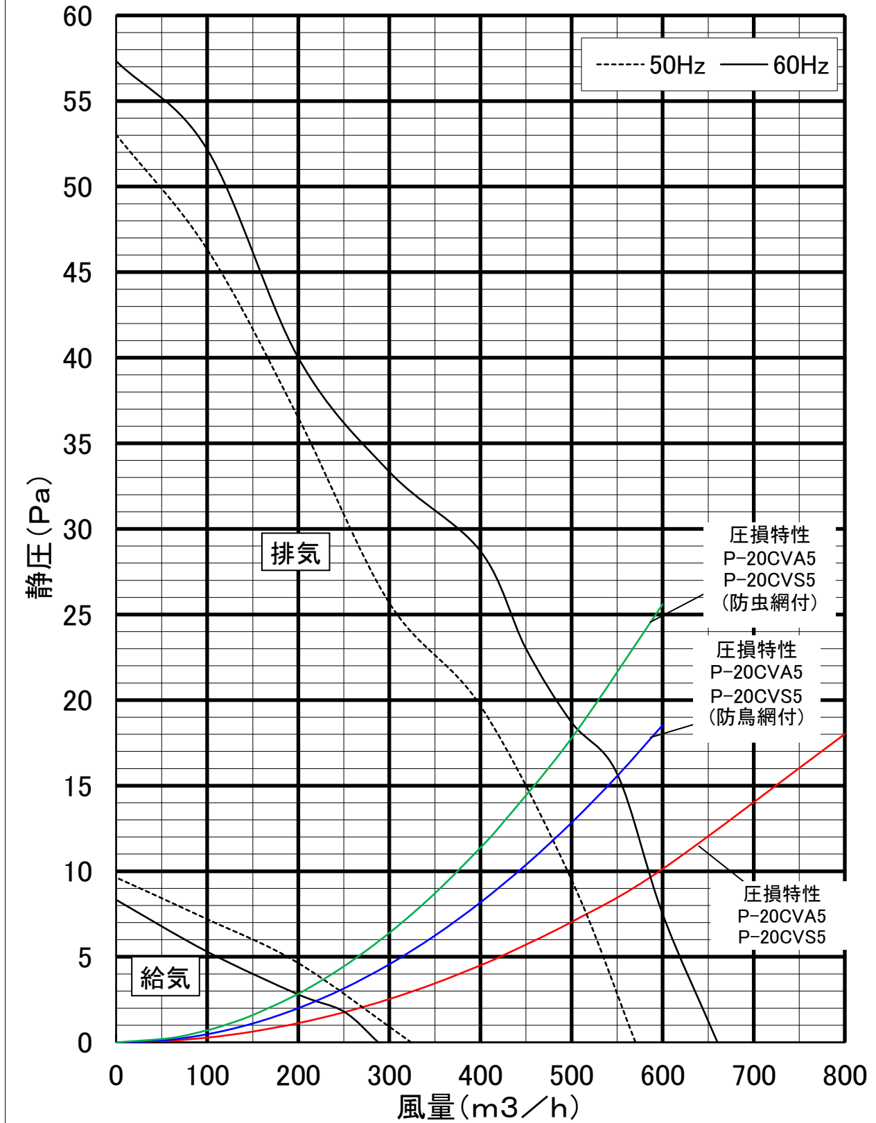
P-Q曲線
