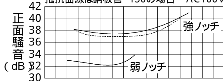
抵抗曲線は鋼板管 150の場合 AC100V
