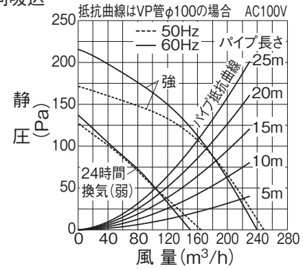
3方向吸込
