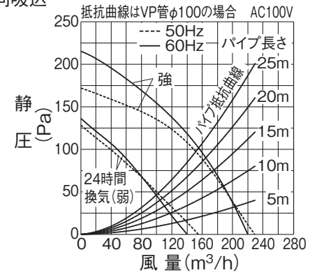
2方向吸込
