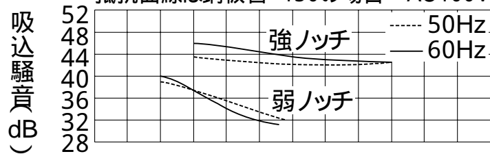
抵抗曲線は鋼板管 150の場合 AC100V
