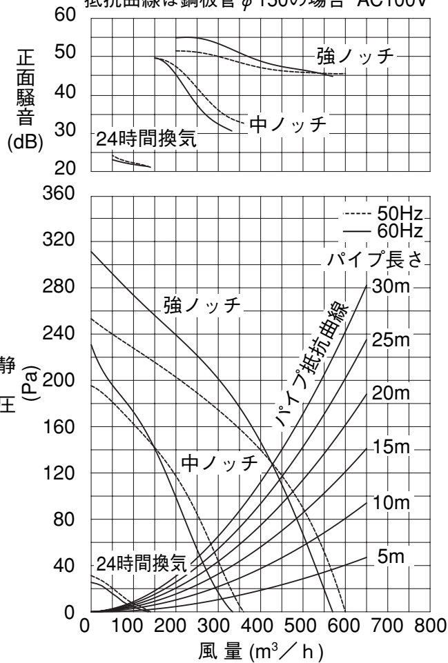
抵抗曲線は銅板管 \phi 150 の場合 AC100V
