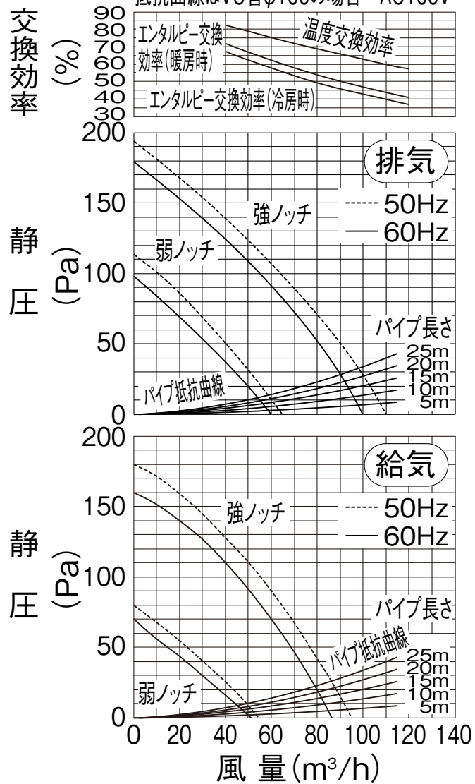
抵抗曲線はVU管φ100の場合 AC100V
