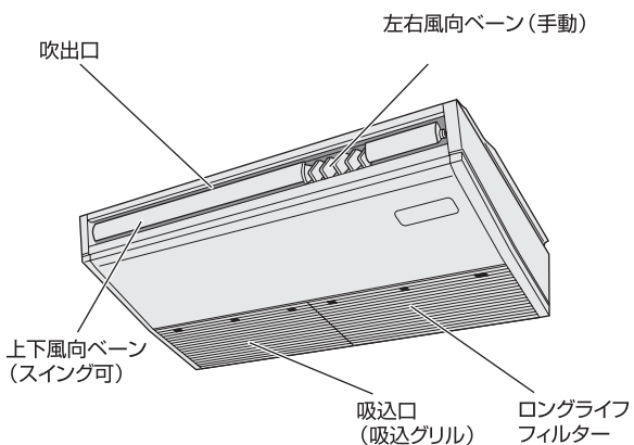
PCFY-KM形 天吊形
