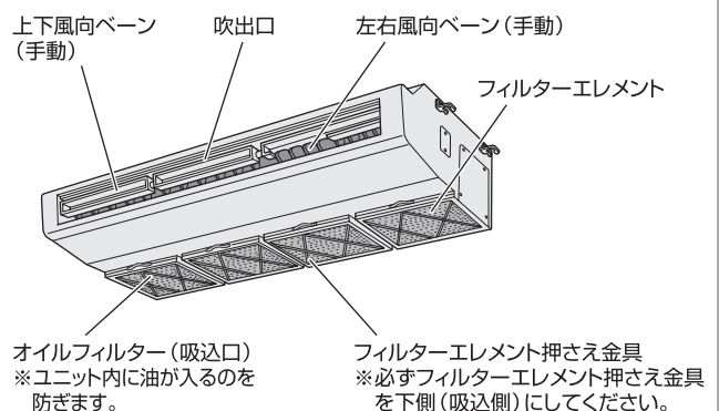
PCFY-HM形 厨房用天吊形
