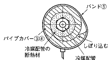
接続部断面
