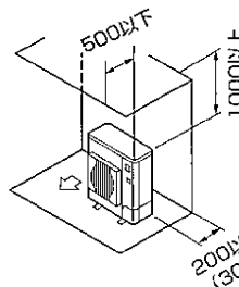
(2) 背面と上方に障害物がある場合 (正面、側面は開放)
