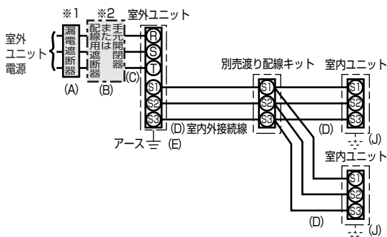
—同時ツインシステムの配線—
