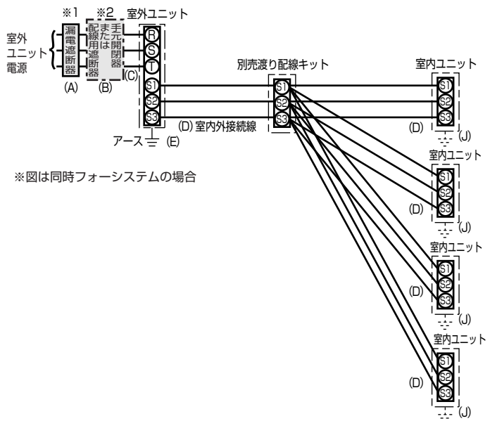
—同時トリプル・フォーシシステムの配線—
