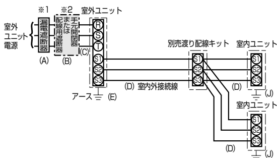
—同時ツインシステムの配線—
