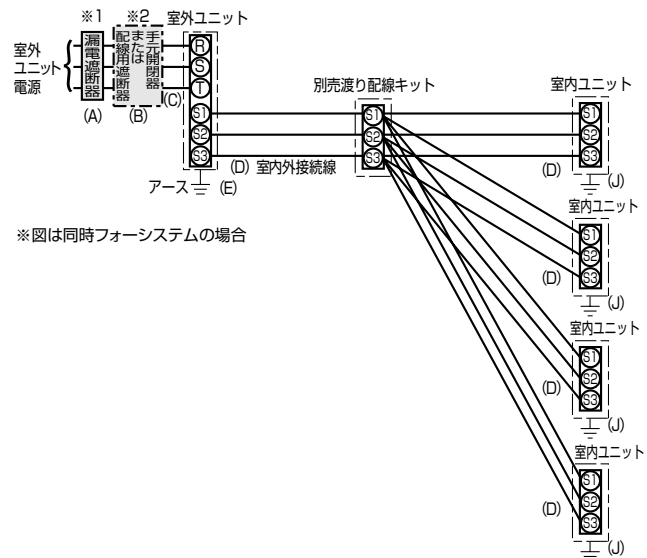
—同時トリプル・フォーシステムの配線—
