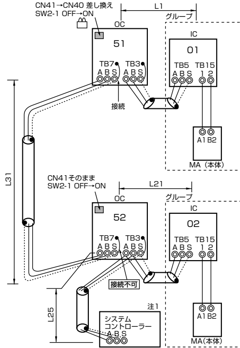
制御線配線例
