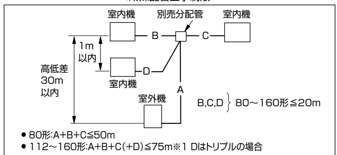
<冷媒配管工事制限>
