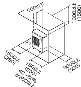
(6) 背面と側面および上方に障害物がある場合 (正面は開放)
