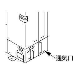
ERMP CRMP112~160形の場合
